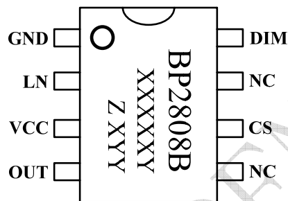
图 2 管脚封装图
