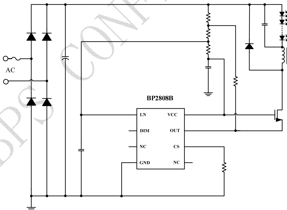
图 1 典型应用图
