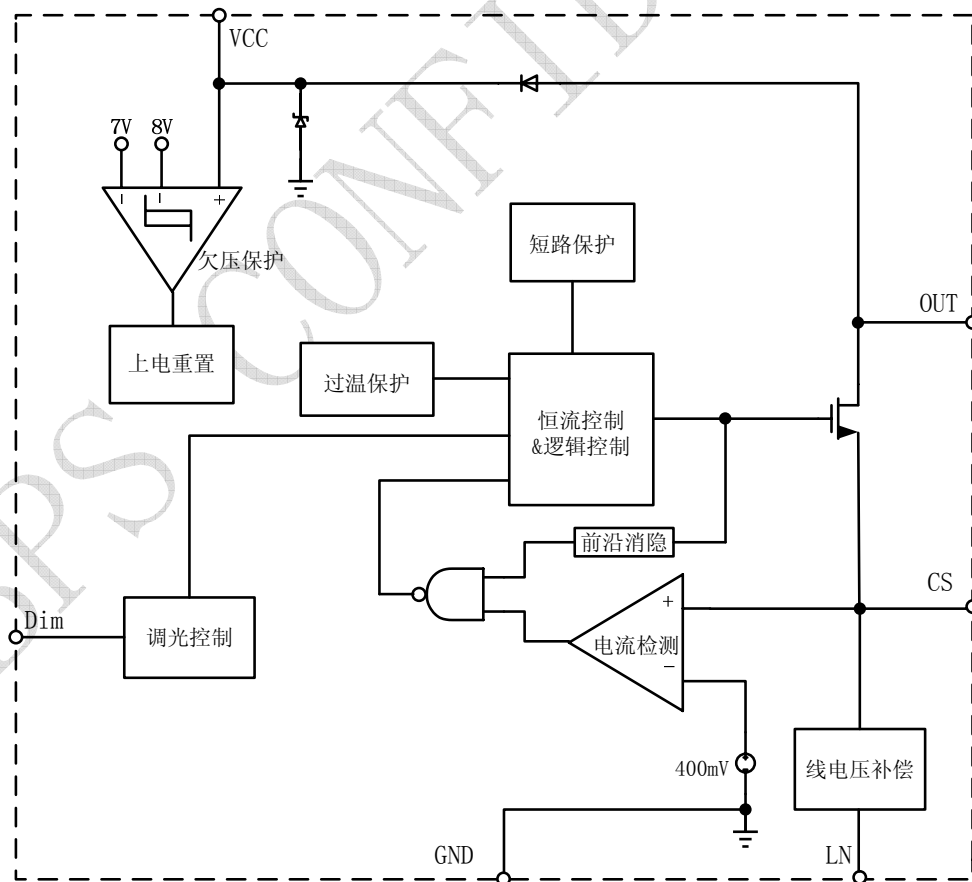
图 3 BP2808B 内部框图
