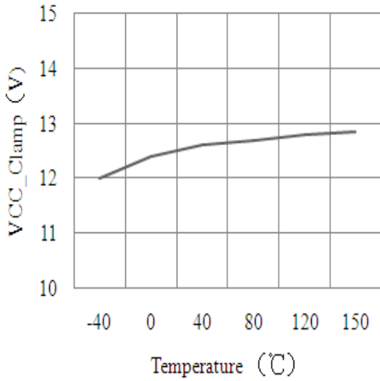
V CC 钳位电压对温度的变化
