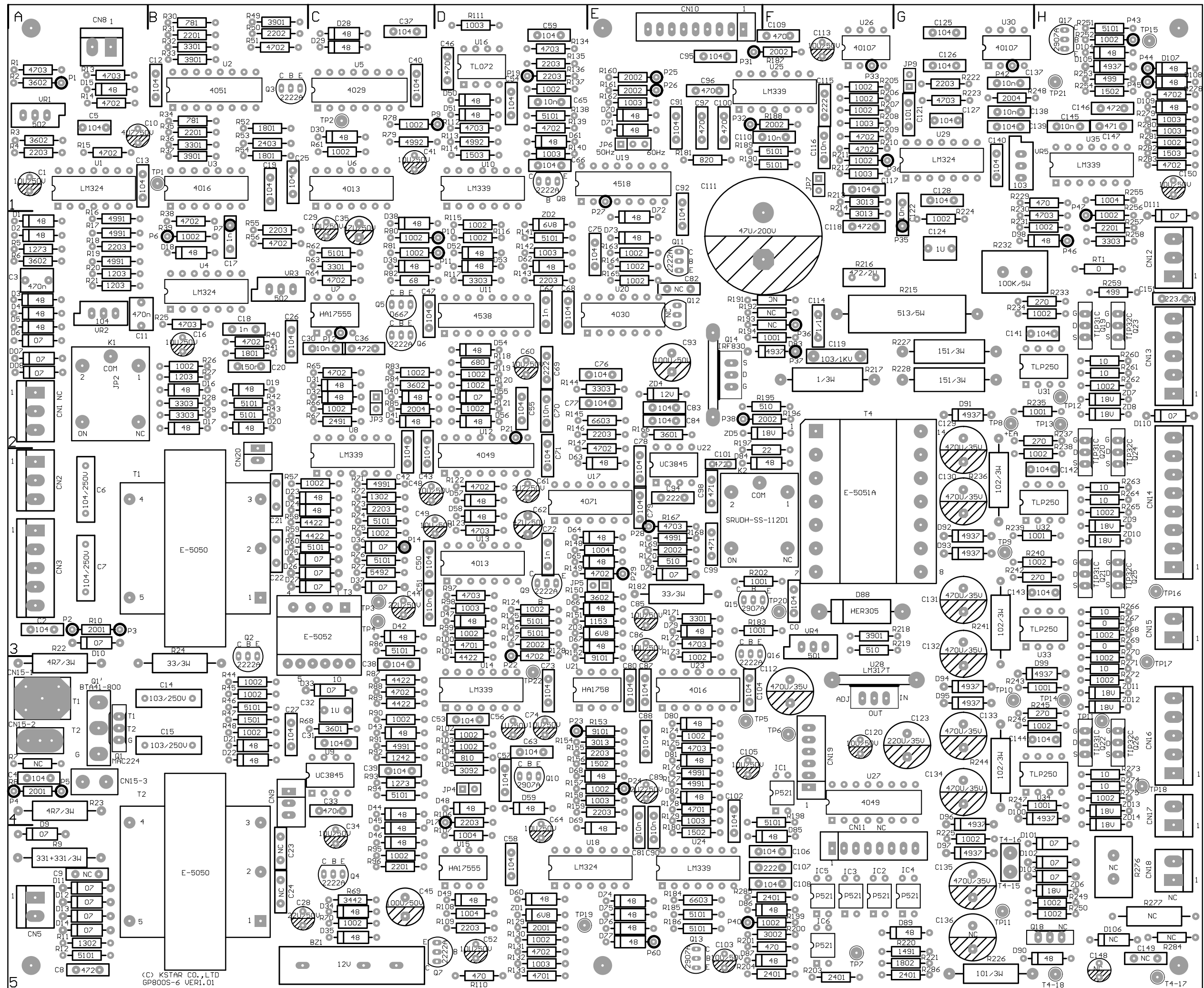
图12.2 KSTAR-GP802型工频机主板布局图
