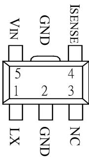
T6322A-DXG SOT-89-5
