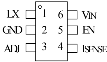
T6322A-AXG SOT-23-6
