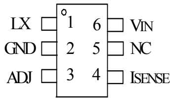
T6322A-CXG SOT-23-6
