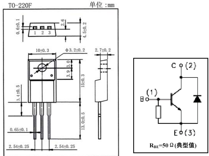
引脚： 1. B 2. C 3. E
