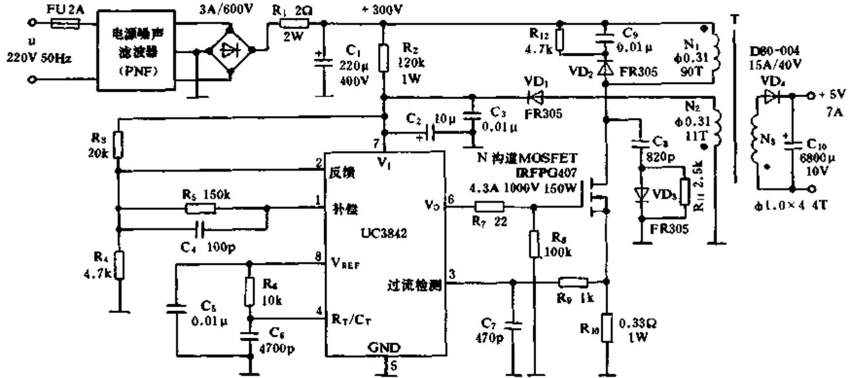
图 9.3.3 UC3842 的典型应用电路
