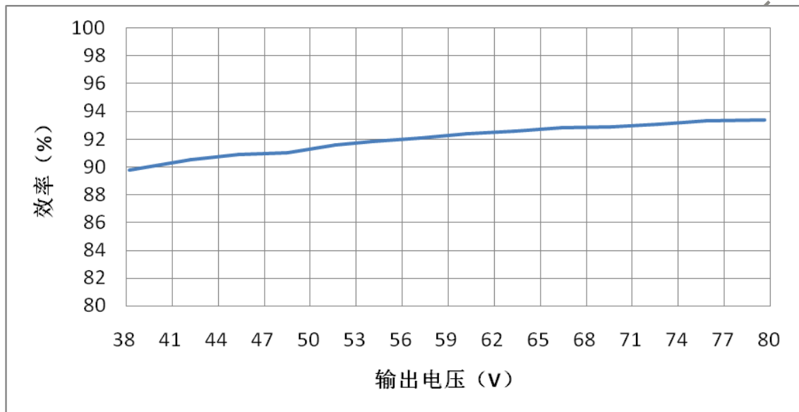
效率对负载的曲线图
