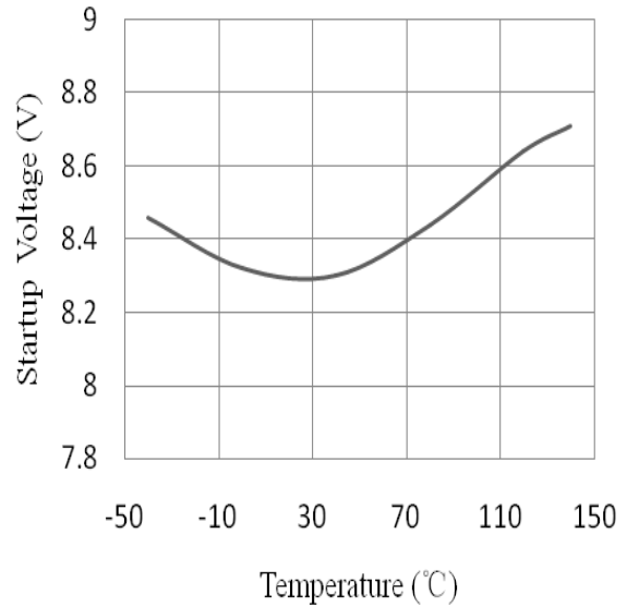
启动电压对温度的变化
