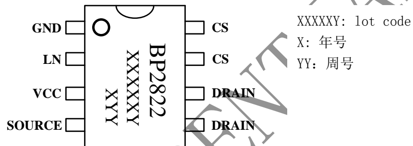
图 2 管脚封装图
