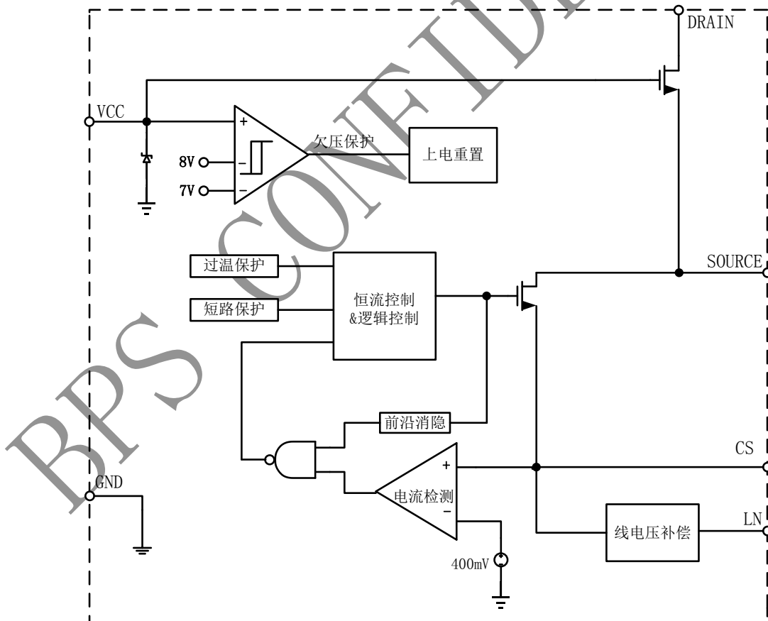
图 3 BP2822 内部框图
