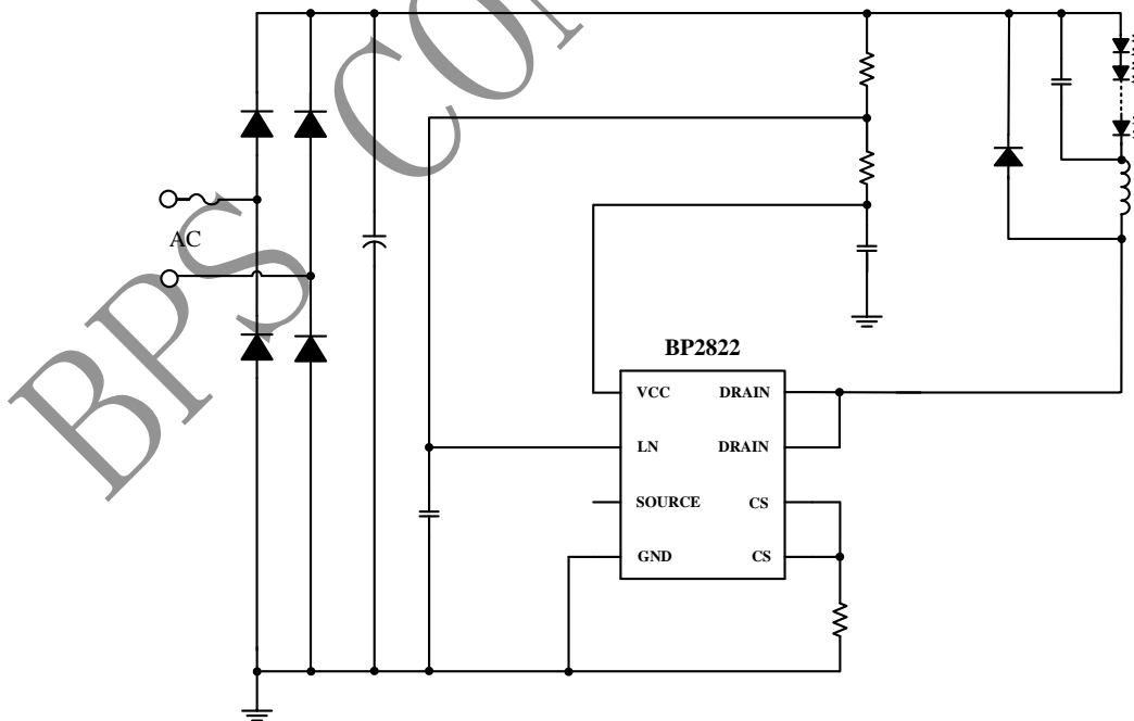
图 1 典型应用图
