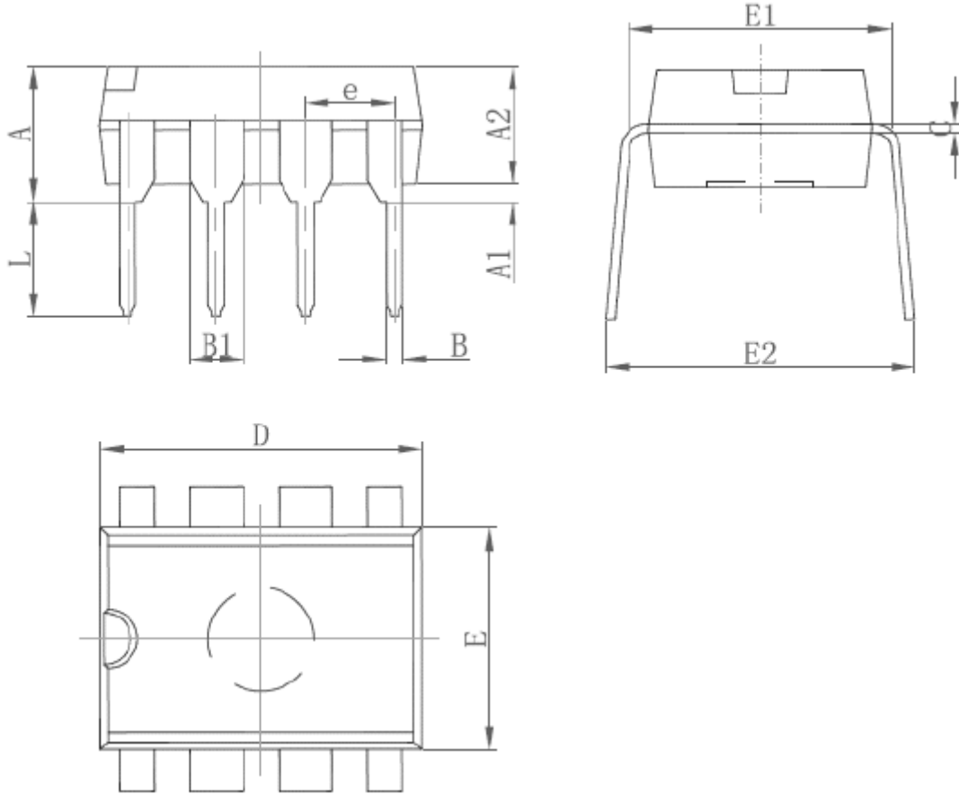
DIP8 封装外观图
