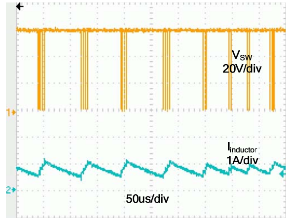
输出负载短路后
