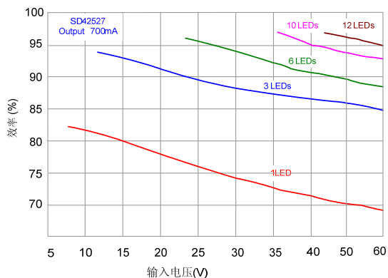
输出 700mA 效率随输入电压变化曲线
