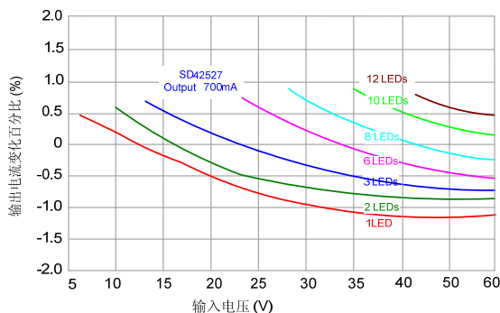
输出 700mA 电流随输入电压变化率
