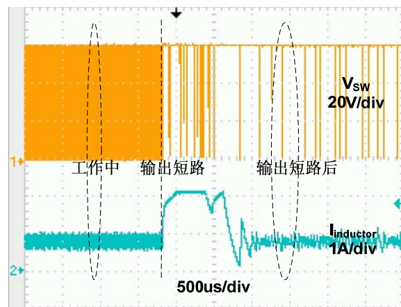
工作 -> 输出负载短路
