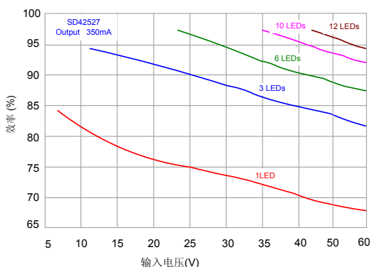
输出 350mA 效率随输入电压变化曲线
