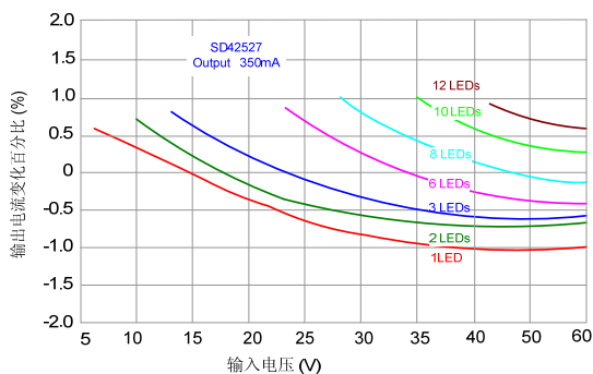
输出 350mA 电流随输入电压变化率
