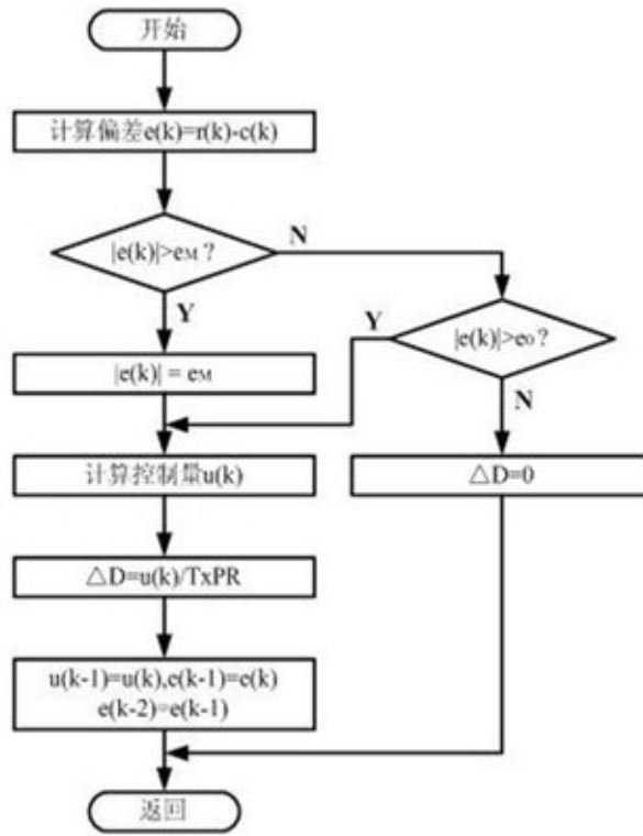
图 4-10 PID 调节子程序流程图
