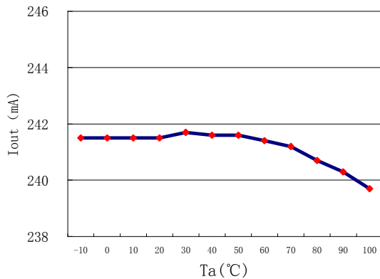
c) 环境温度对输出电流曲线图
