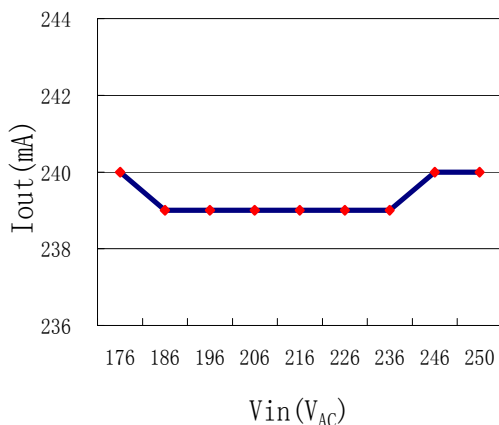
c) 输入电压对输出电流曲线图
