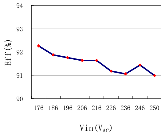
d) 输入电压对系统效率曲线图
