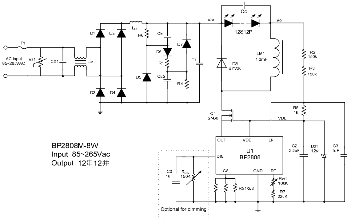
图表 2 交流全电压输入典型应用原理图
