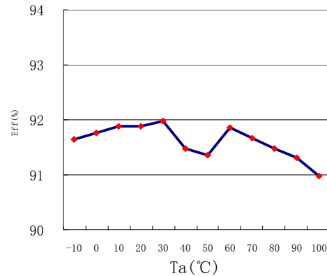
d) 环境温度对系统效率曲线图
