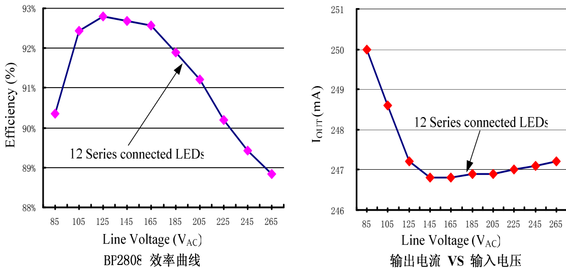
图表 1 效率和恒流特性
