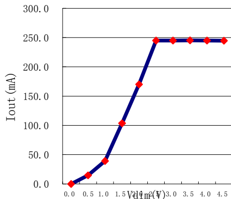
a) Vdim 对输出电流曲线图
