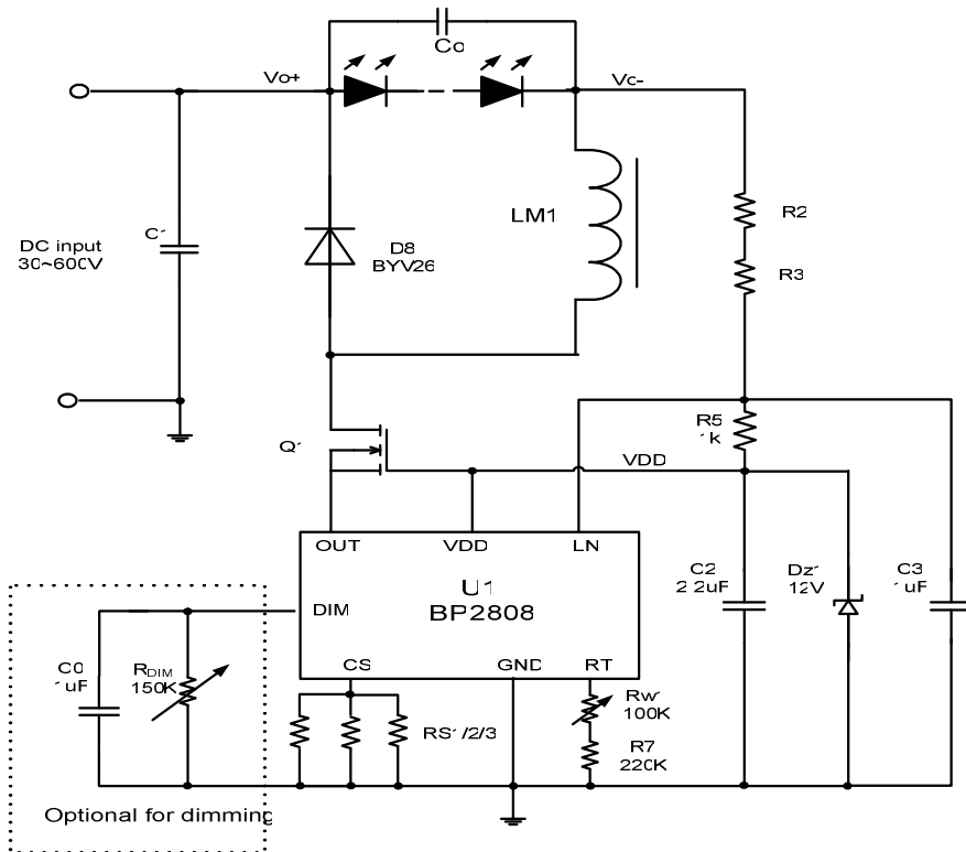
图表 3 直流输入典型应用原理图
