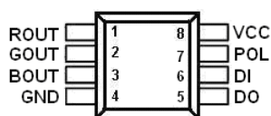
Fig1 SOP-8 封装
