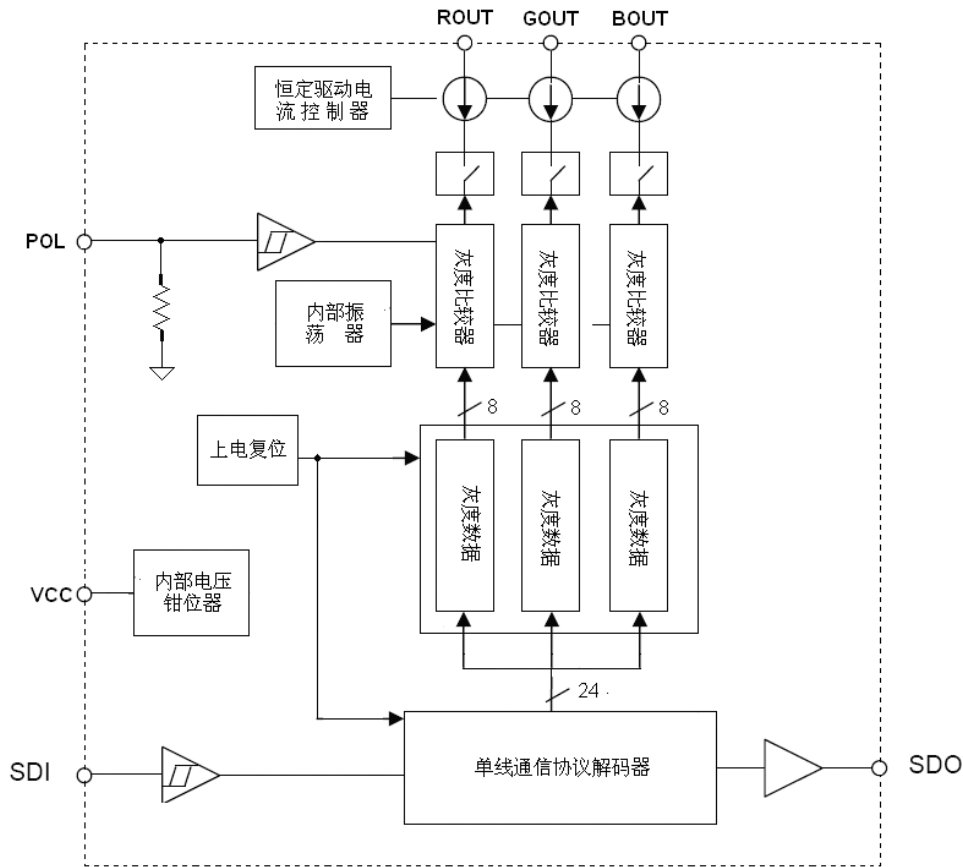
电路内部框图
