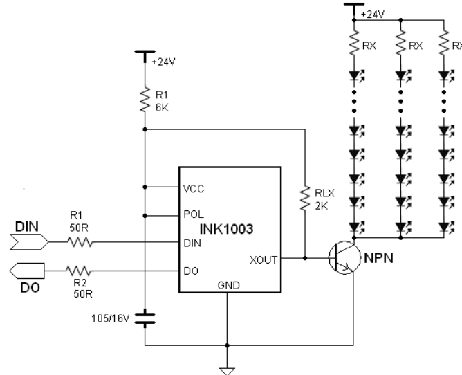
Fig6, 典型高压恒压应用
