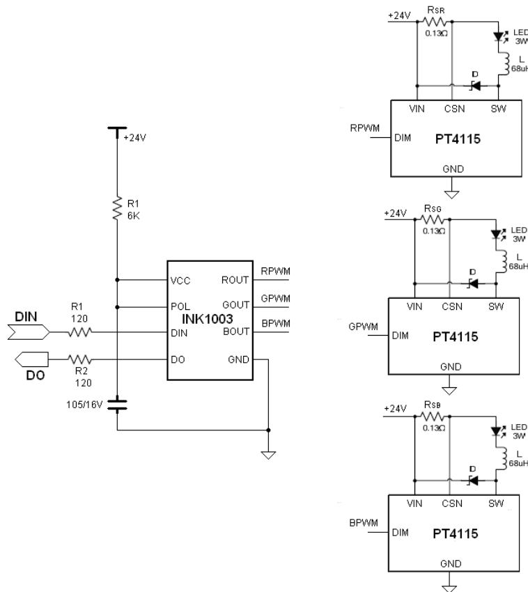
Fig6, 典型大功率恒流应用
