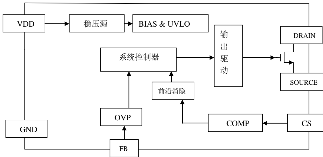
图 1 R8121 功能框图
