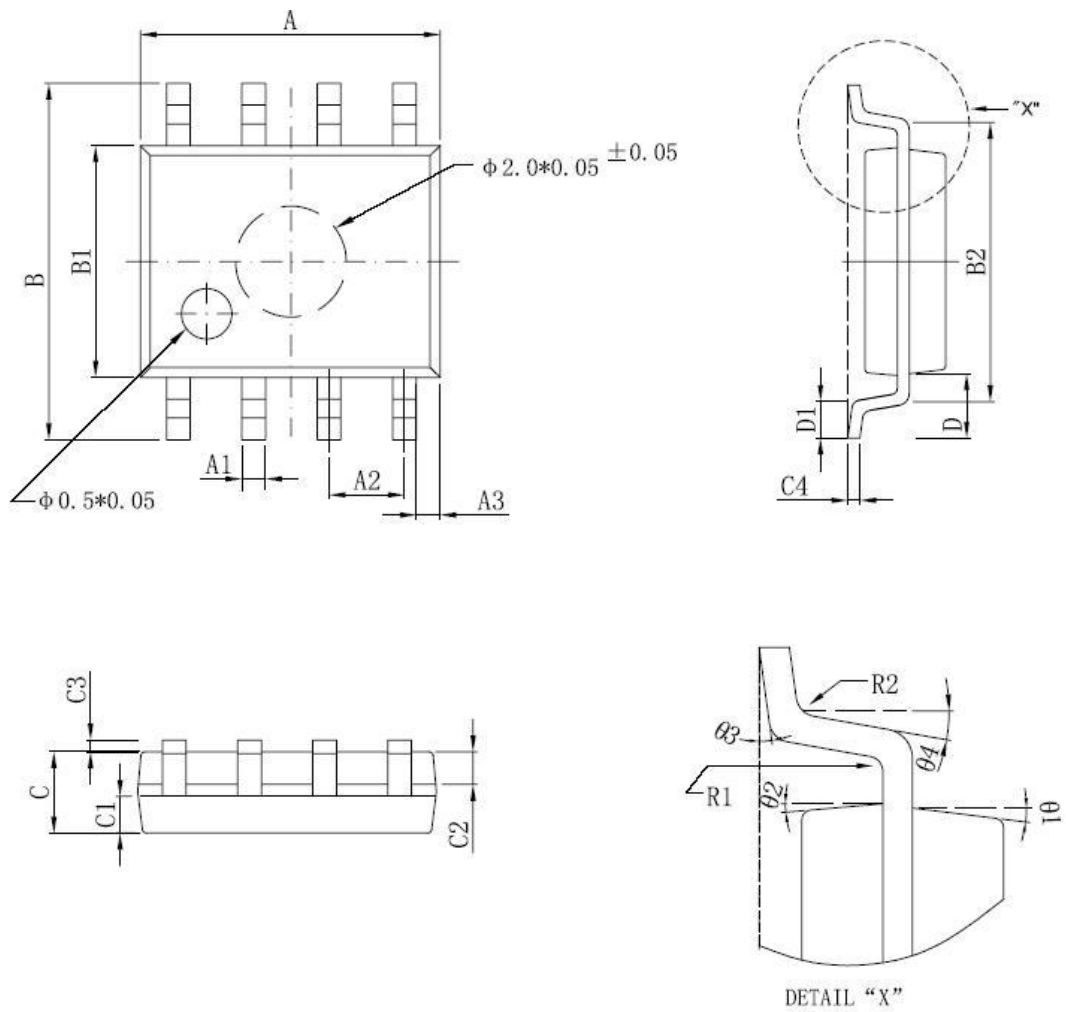
SOP8 封装外形图及尺寸 (R8121CF)
