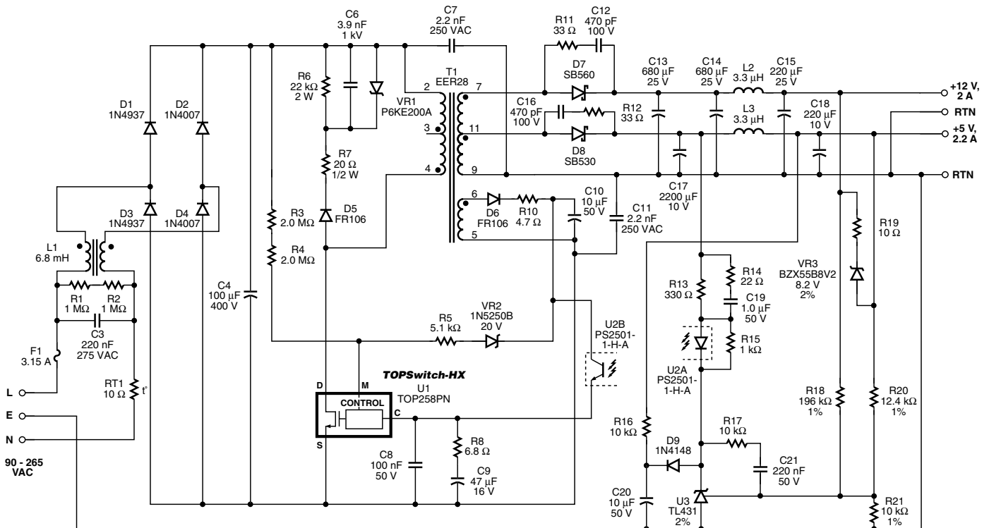
图 1. 通用输入、35 W输出的LCD电源，使用TOP258PN器件
