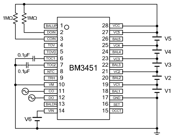
测试电路 3
