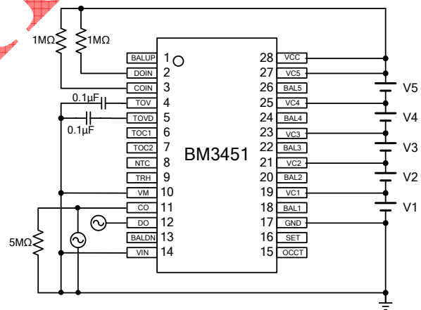
测试电路 2
