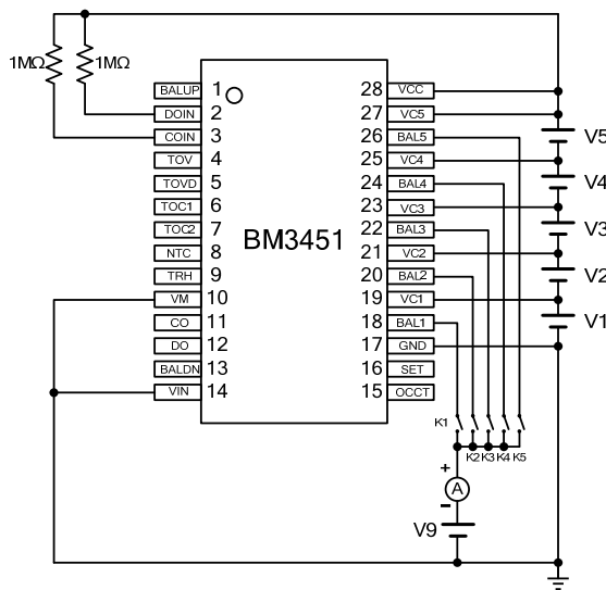
测试电路 8
