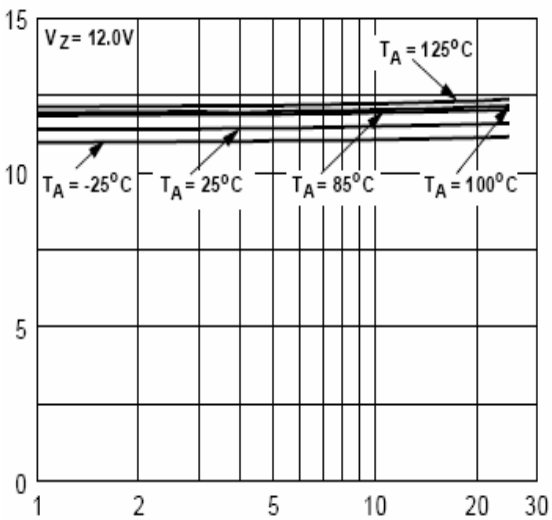
V_Z - I_Z
