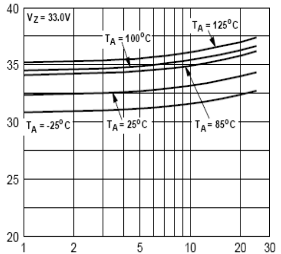
V_Z - I_Z
