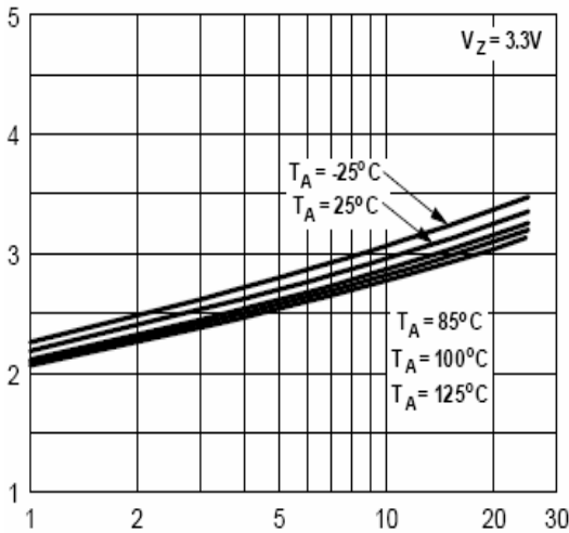
V_Z - I_Z
