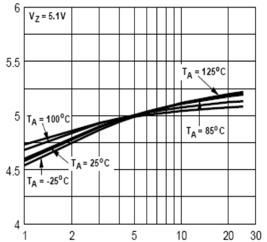
V_Z - I_Z
