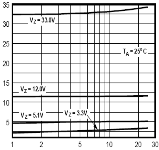
V_Z - I_Z
