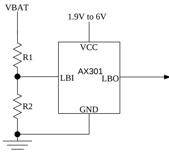
图 2 被监测电池电压高于6V
