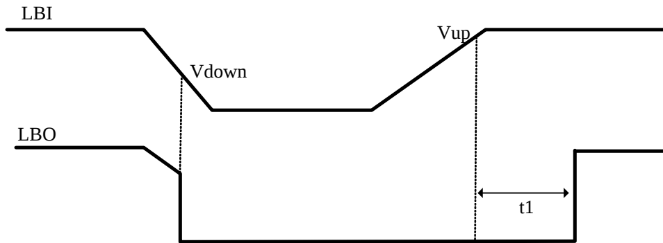
图 3 AX301 的工作时序
