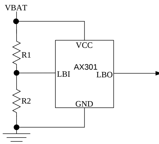
图 1 被监测电池电压低于6V
