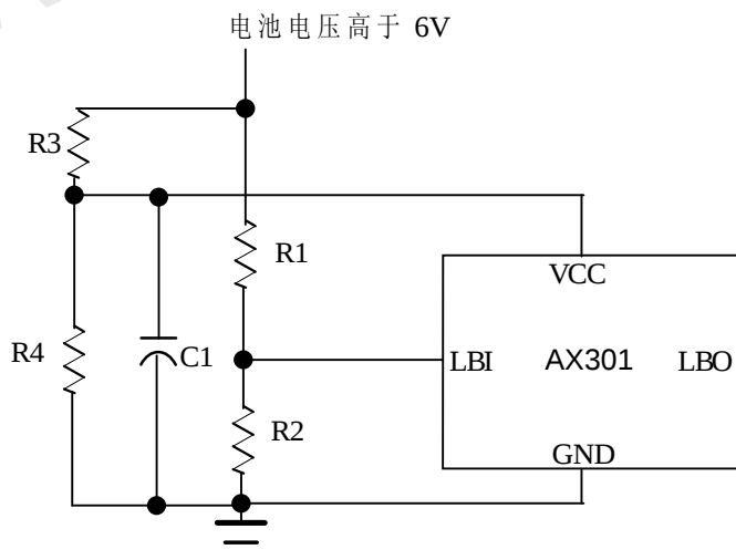
图 9 利用两个电阻分压为AX301供电
