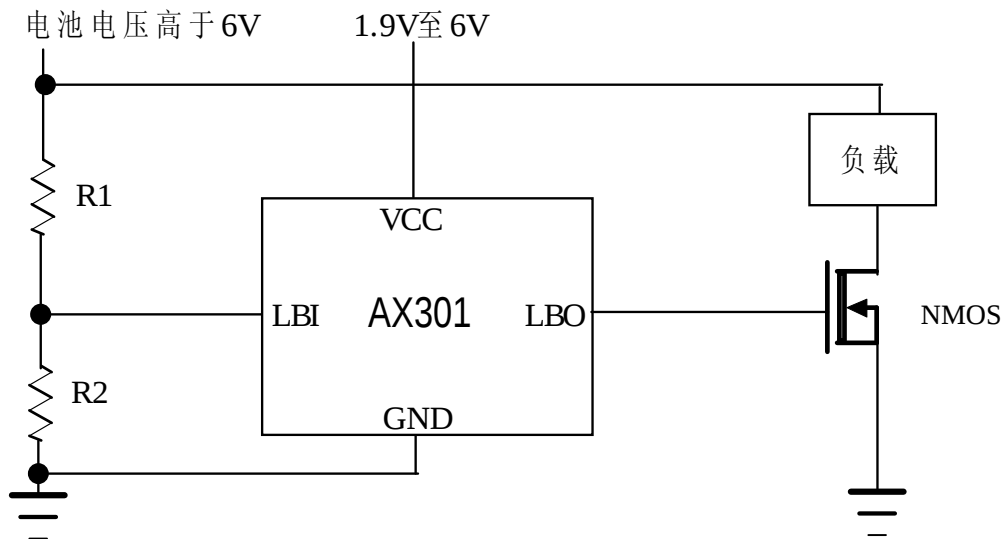
图 6 电池最高电压大于6V，AX301控制NMOS晶体管
