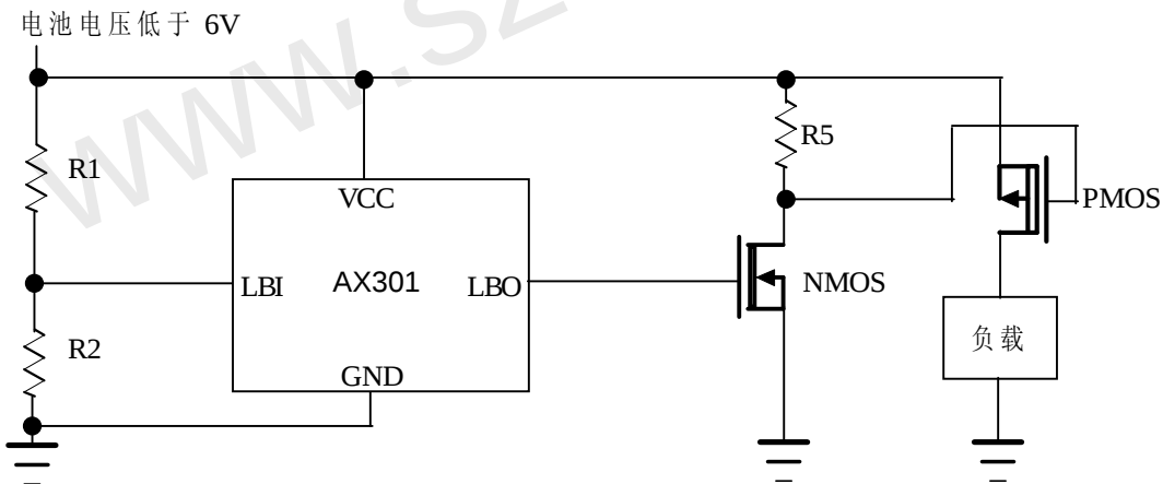
图 7 电池最高电压低于6V，AX301控制PMOS晶体管
