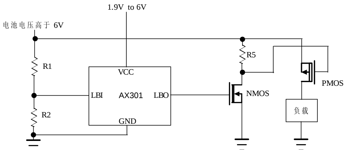
图 8 电池最高电压高于6V，AX301控制PMOS晶体管
