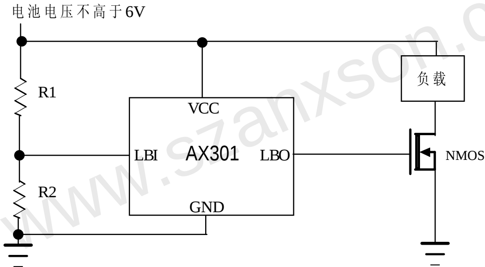
图 5 电池最高电压小于6V，AX301控制NMOS晶体管
