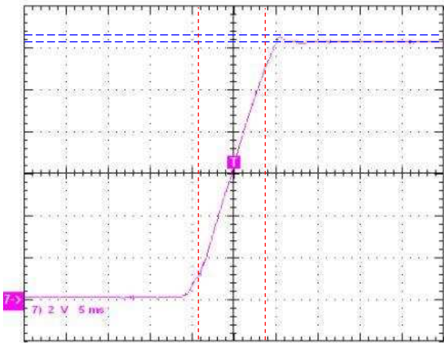
图 12. 输出电压开启, 265Vac, 空载 2V/div 5ms/div
