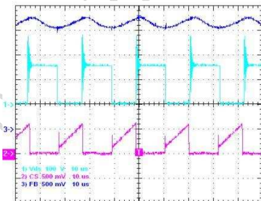
图 22 FB, Vds, Sense 波形, 85Vac, 满载
