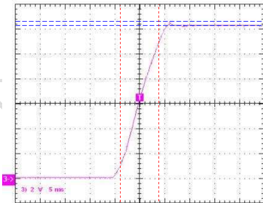
图 9. 输出电压开启, 85Vac, 空载 2V/div 5ms/div
