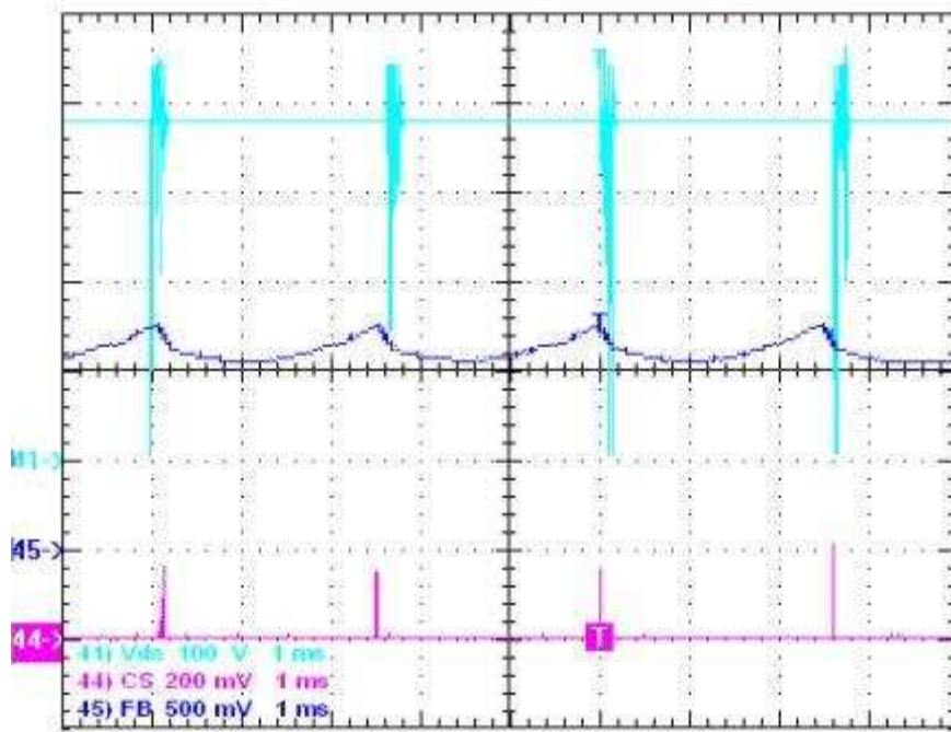
图 25 FB, Vds, Sense 波形, 265Vac, 空载
