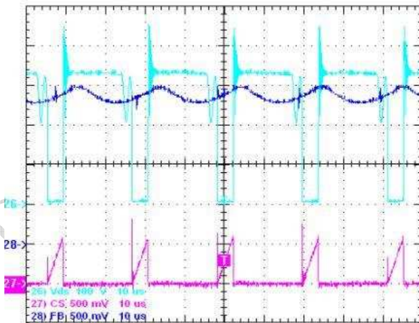
图 24 FB, Vds, Sense 波形, 180Vac, 满载
