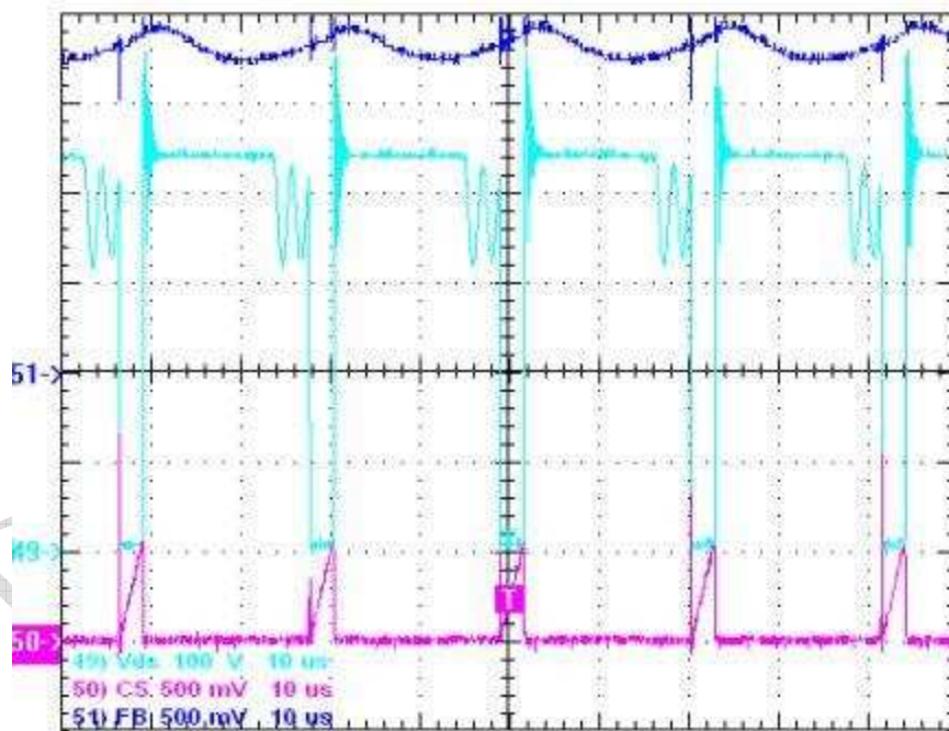
图 26 FB, Vds, Sense 波形, 265Vac, 满载
