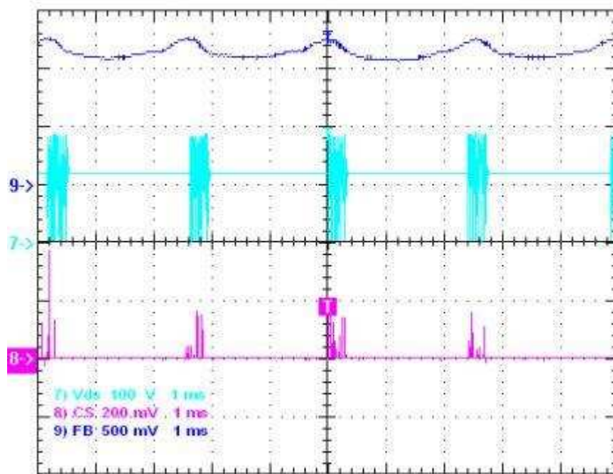
图 21 FB, Vds, Sense 波形, 85Vac, 空载
