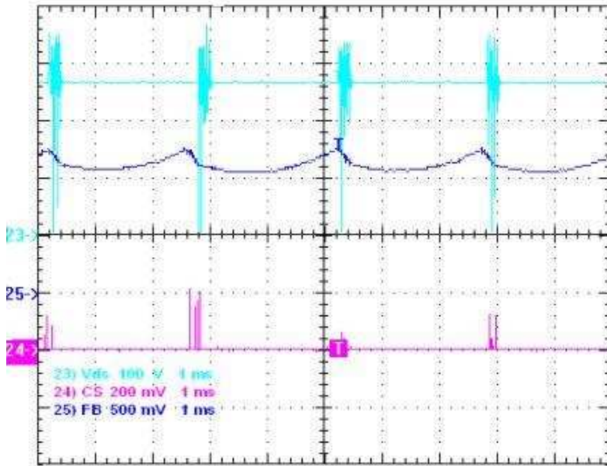
图 23 FB, Vds, Sense 波形, 180Vac, 空载
