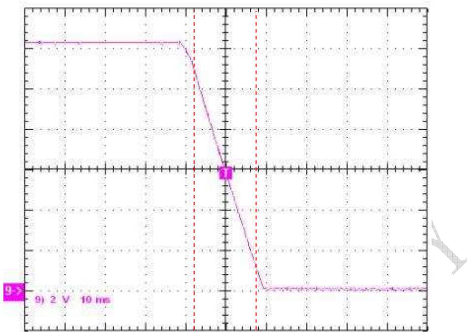
图 14. 输出电压关断, 265Vac, 满载 2V/div 10ms/div
