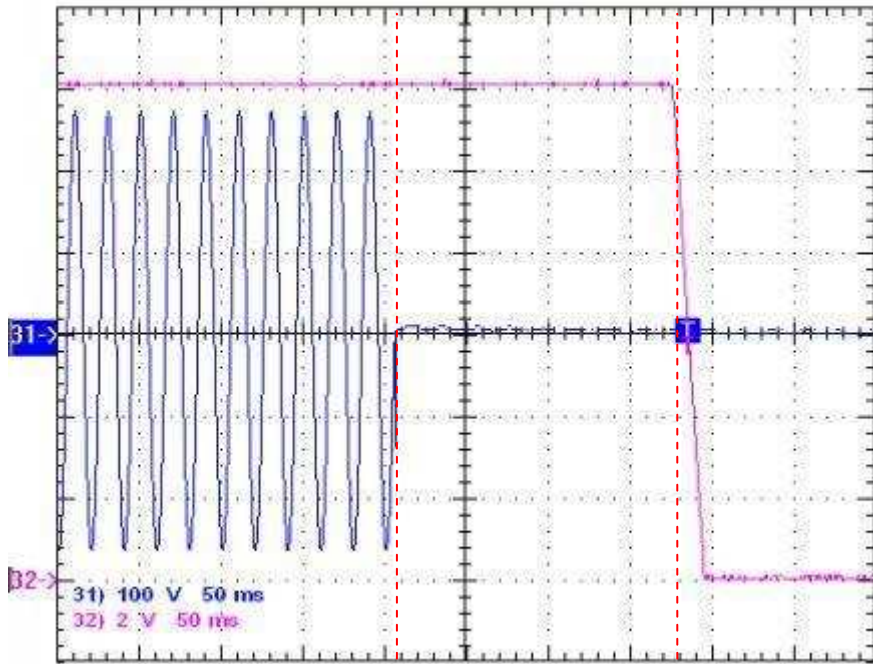
图 20. 关断保持时间，265Vac 满载
