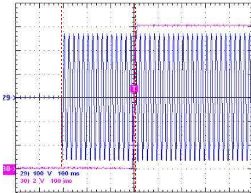
图 18. 启动延迟, 265Vac 满载
