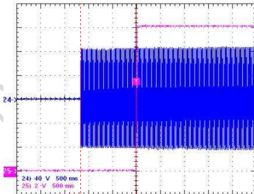
图 17. 启动延迟, 85Vac 满载
