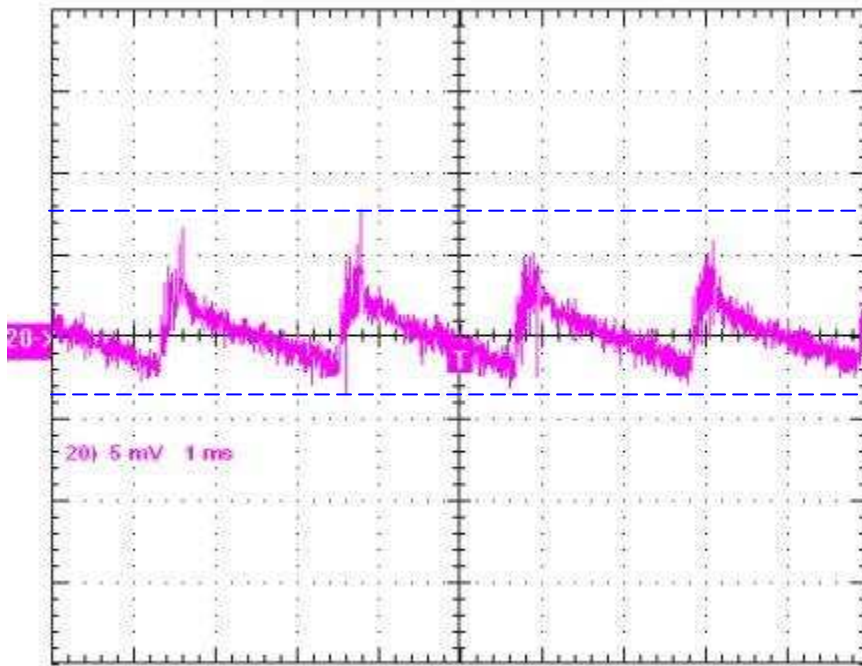
图 3 纹波噪声波形, 180Vac, 空载 5mv/div 1ms/div
