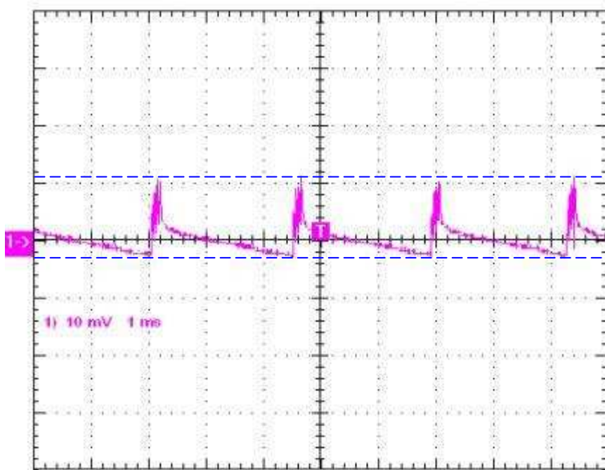
图7 纹波噪声波形, 265Vac, 空载 10mV/div 1ms/div
