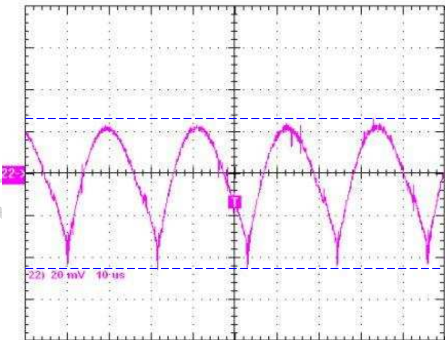
图 6 纹波噪声波形, 230Vac, 满载 20mV/div 10us/div
