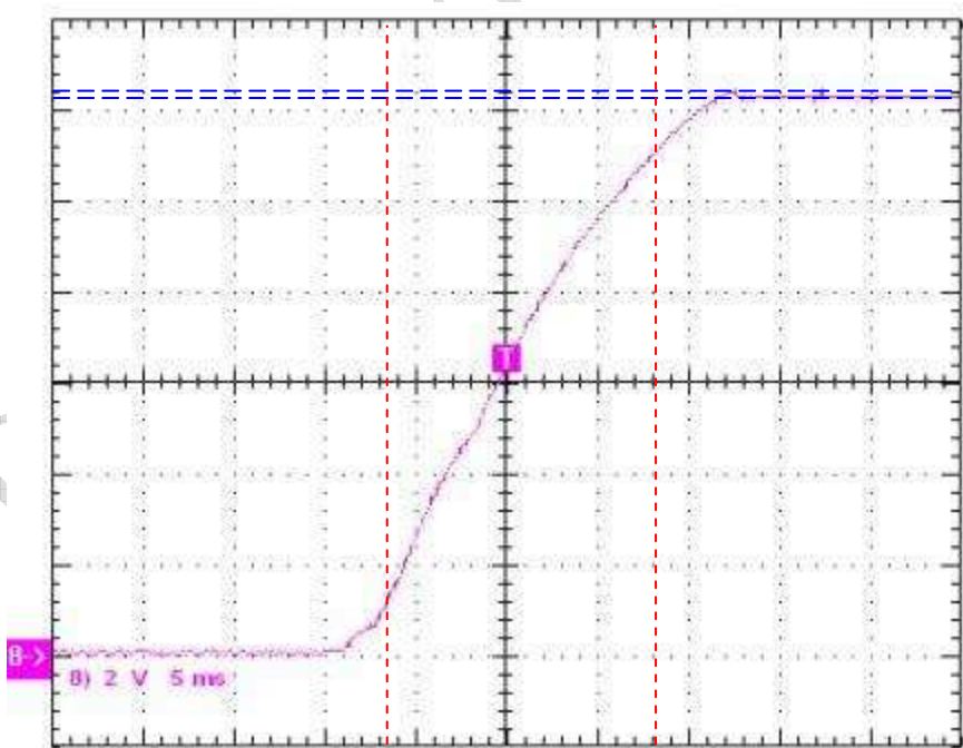
图 13. 输出电压开启, 265Vac, 满载 2V/div 5ms/div
