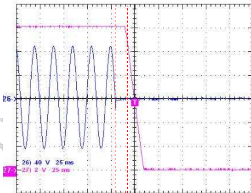
图 19. 关断保持时间, 85Vac 满载
