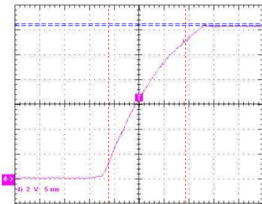
图 10. 输出电压开启, 85Vac, 满载 2V/div 5ms/div
