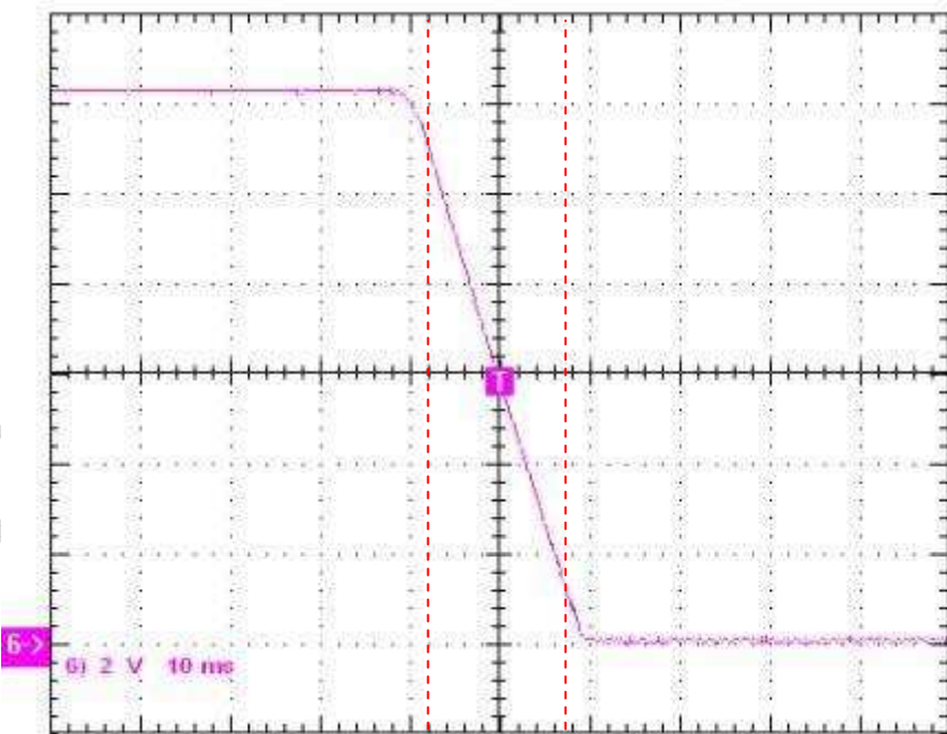
图 11. 输出电压关断, 85Vac, 满载 2V/div 10ms/div
