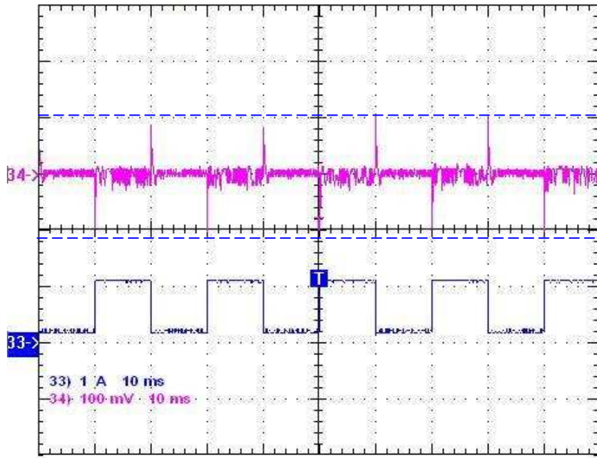
图 15. 动态测试, 85Vac
