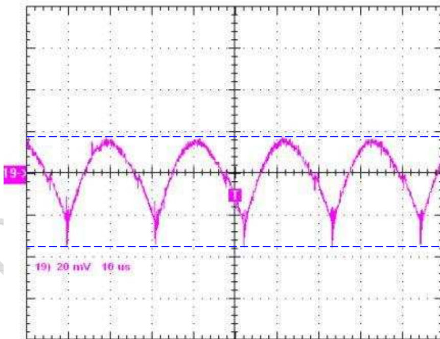
图 4 纹波噪声波形, 265Vac, 满载 20mV/div 10us/div
