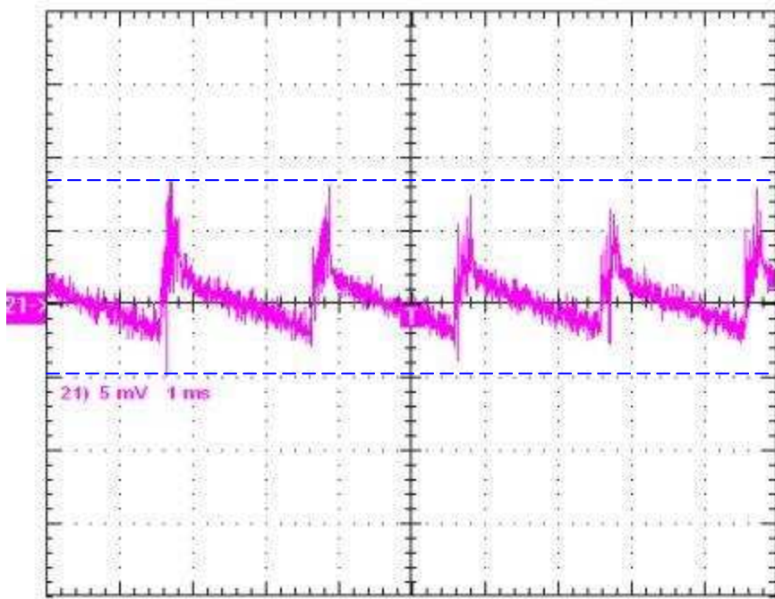
图 5 纹波噪声波形, 230Vac, 空载 5mV/div 1ms/div
