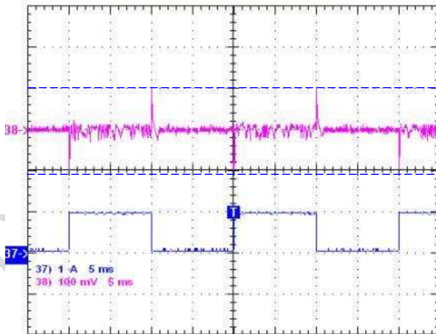
图 16. 动态测试, 265Vac
