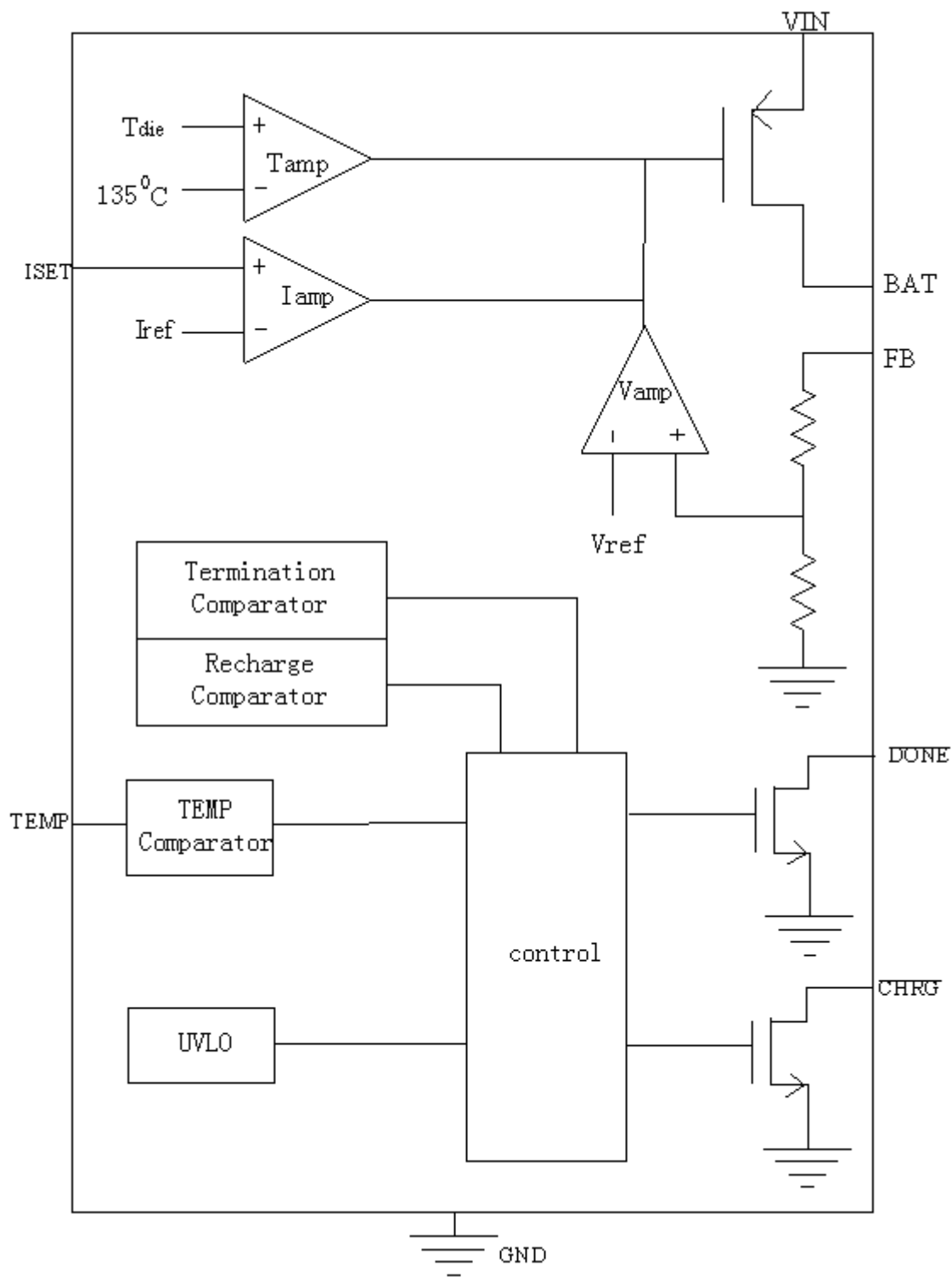
图 3 功能框图
