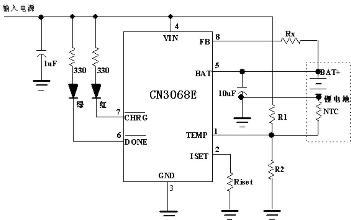
图 1 典型应用电路（恒压充电电压 4.2V）
