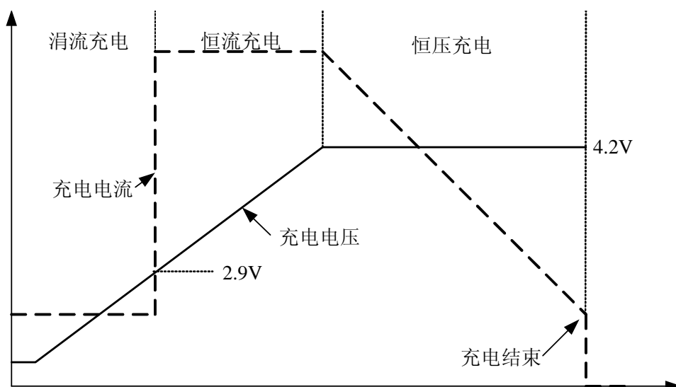
图4 充电过程示意图
