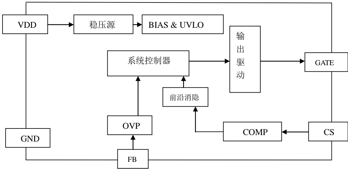
图 1 R8021 功能框图
