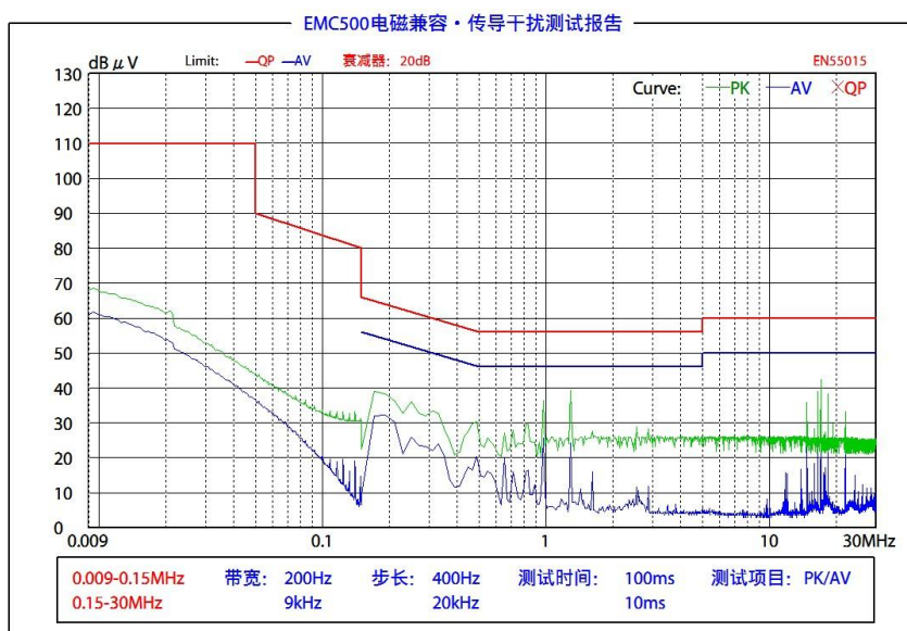
图 1. 传导测试
