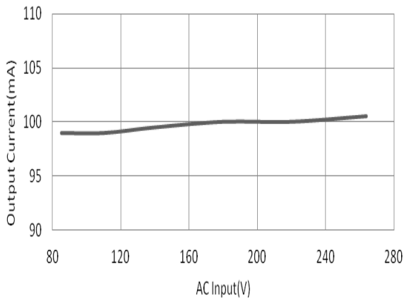
线性调整率
