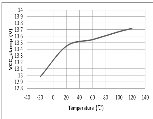
钳位电压对温度的变化
