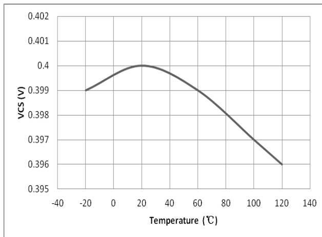
电流检测门限对温度的变化
