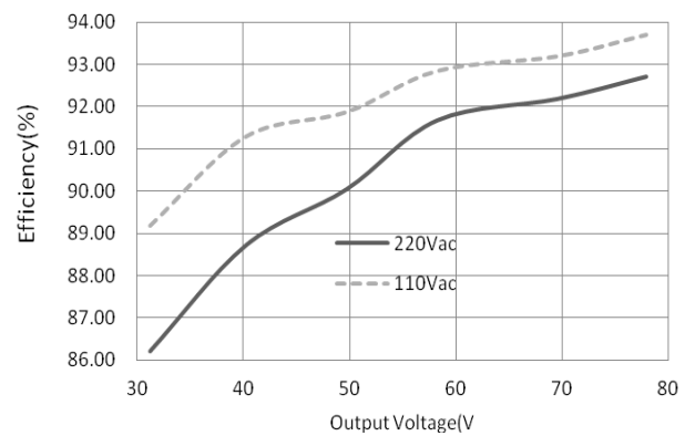
效率对负载的变化
