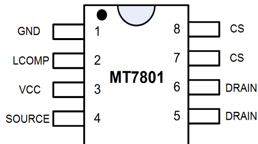
(SOP8)
