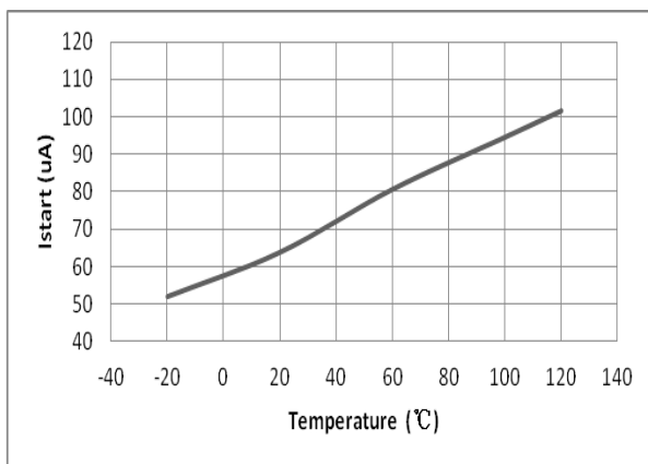
启动电流对温度的变化
