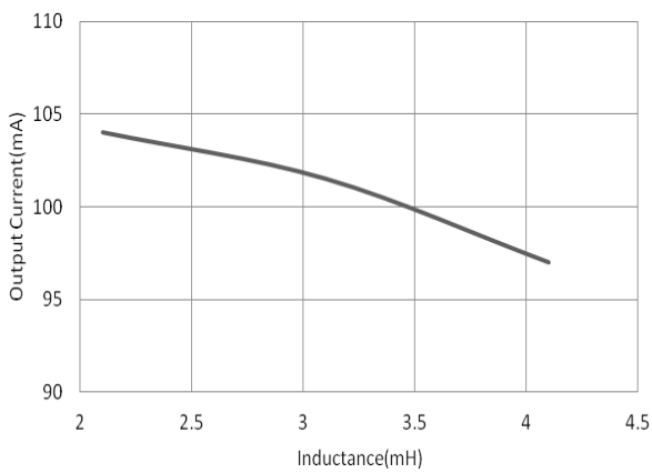
输出电流对电感量的变化
