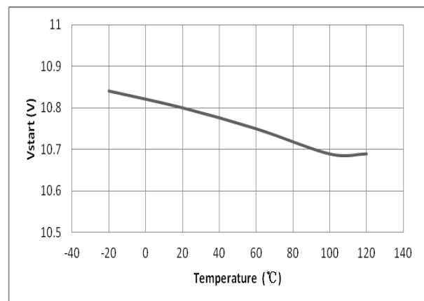
启动电压对温度的变化
