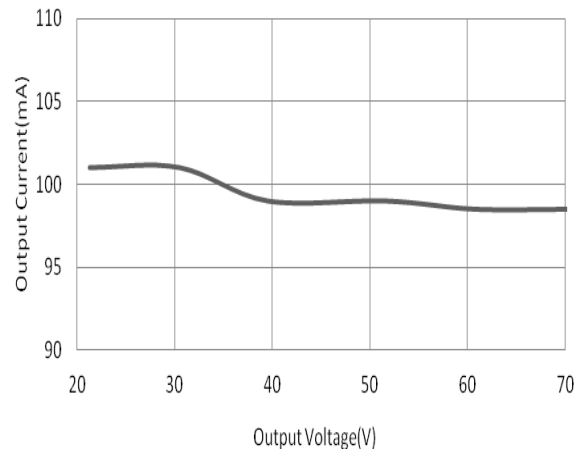
负载调整率
