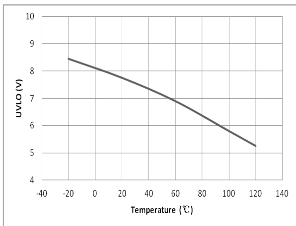
欠压保护门限对温度的变化
