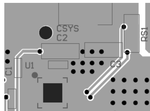
Bottom Layer
