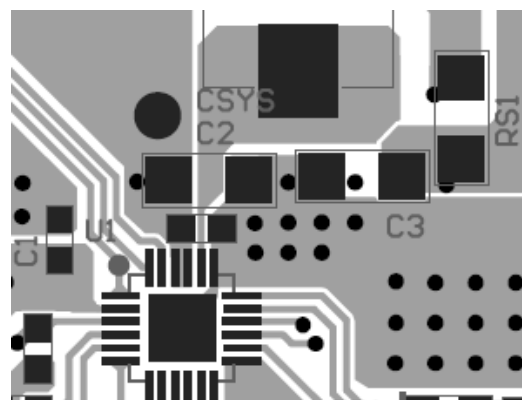
Top Layer
