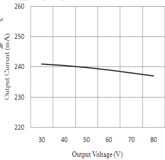
负载调整率
