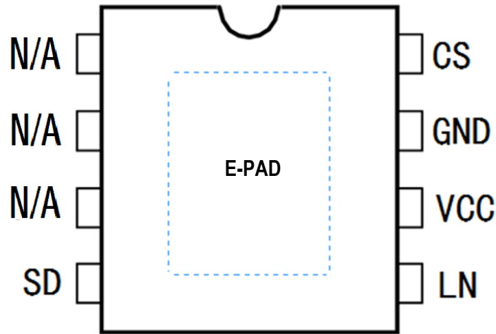
ESOP8 封装
