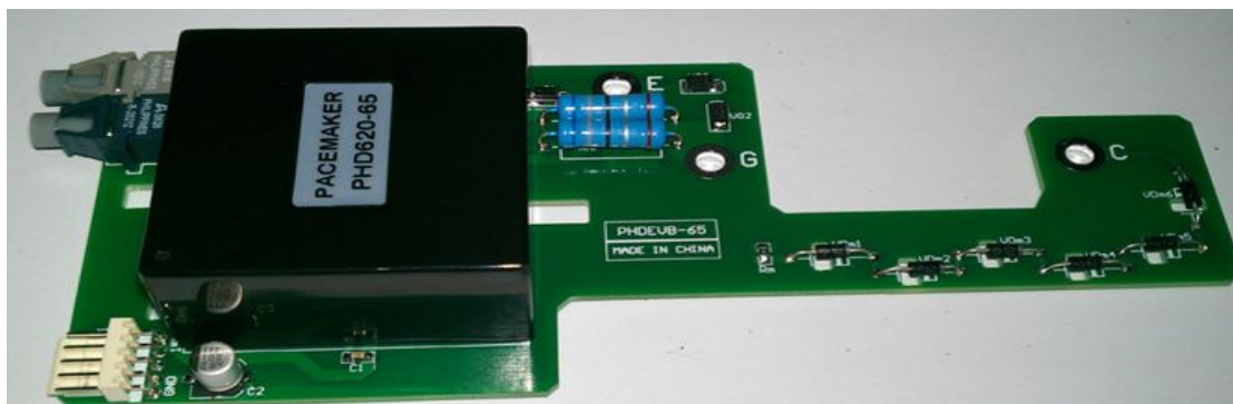
图 3b PHVDREVB65-X 高压驱动板相片
