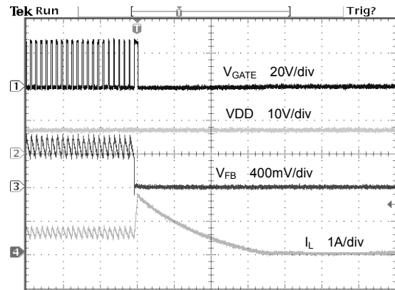
t-100µs/div
