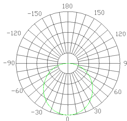
配光曲线
