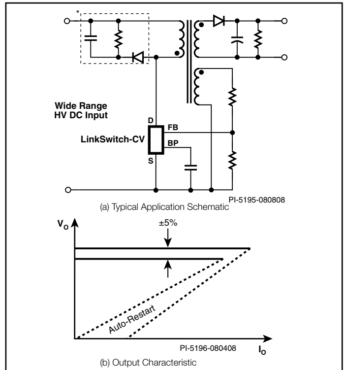
图1. 典型应用电路图(a)及输出特性包络(b) *可选用LNK623-624PG/DG。(有关引脚及其他外部电路设计的注意事项，请参阅“主要应用指南”部分)
