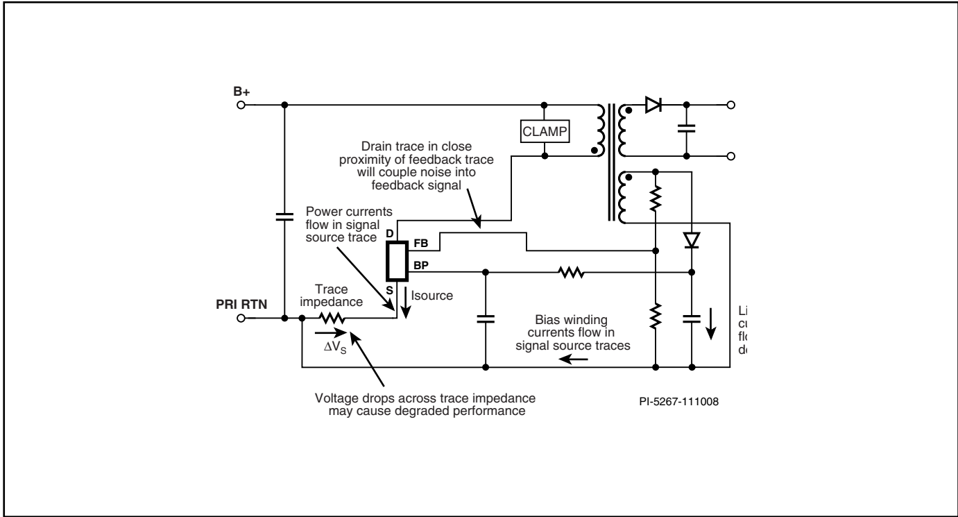
图8. 不合理布局的电气影响电路图示
