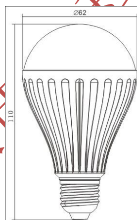
产品尺寸 (单位 mm)
