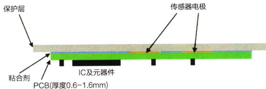
图1 基于两层板的电容式触摸模组的结构
