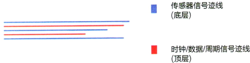
图4 传感器信号迹线和周期信号迹线相邻时平行布设
