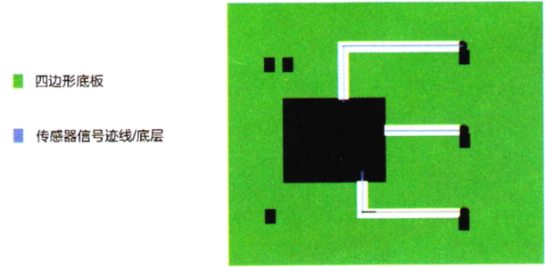
图 2.2 两层PCB板的底层
