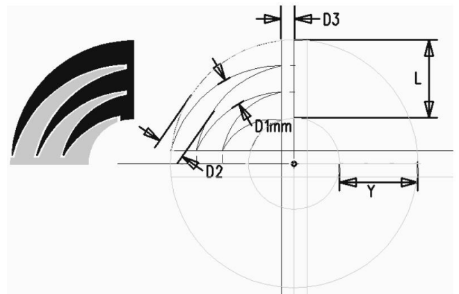
图 10 比例计量触摸转轮设计图
