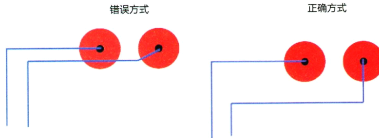
图3 触摸极板下的传感器信号迹线走线方式
