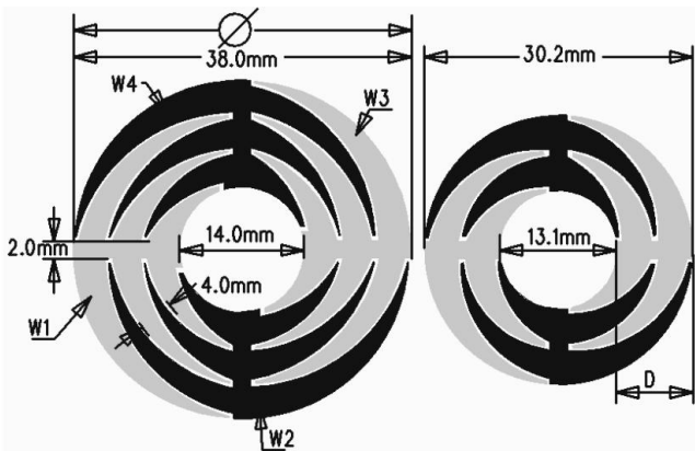
图 9 4 通道比例计量触摸转轮示意图
