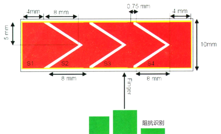
图7 比例计量滑动条的实现
