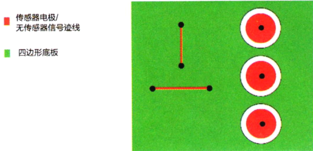
图2.1 两层PCB板的顶层
