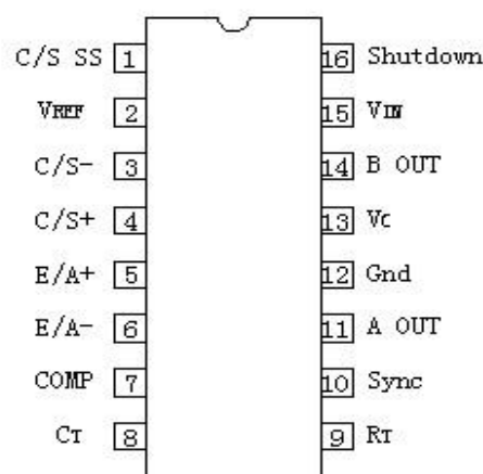
图1-40 UC3846/UC3847 引脚排列
